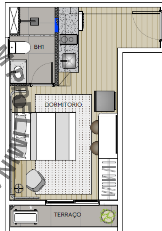
PLANTA TIPO FINAL 09 24m²
